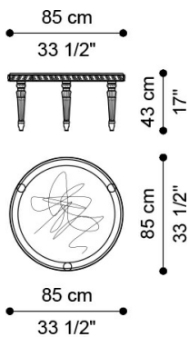
LOW TABLE J.FDL-46B
