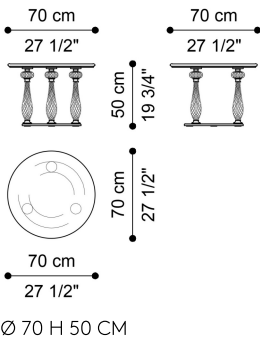
LOW TABLE J.CRYS-56B
